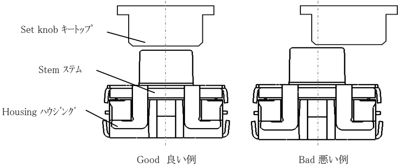
Fig2: Set knob vs stem 図2.キートップとステムの関係
