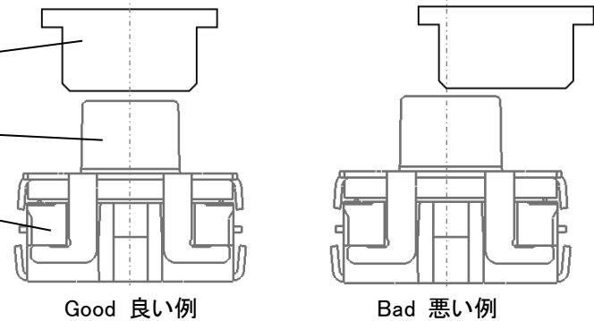
Fig 2: Set knob vs stem 図2: キートップとステムの関係
