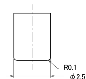
Fig 2: Set knob vs stem 図2: キートップとステムの関係
