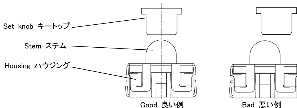
Fig 2: Set knob vs stem 図2: キートップとステムの関係
