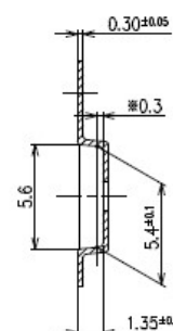
B-B断面図
