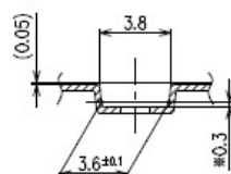
A-A断面图
