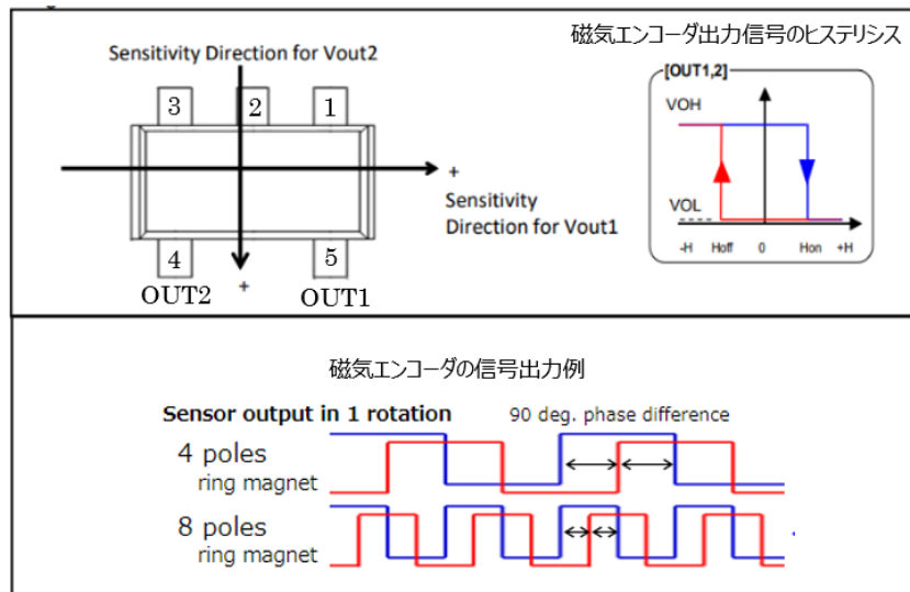
図 9 磁気エンコーダの感度方向と出力
