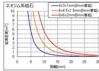
図 2 垂直方向に動作する磁石による磁束密度
