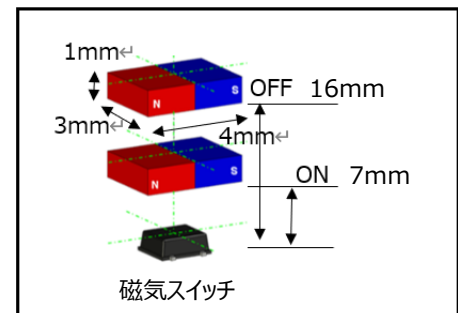
図 4 磁気スイッチと磁石の位置
