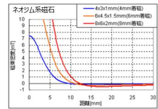
図 3 水平方向に動作する磁石による磁束密度
