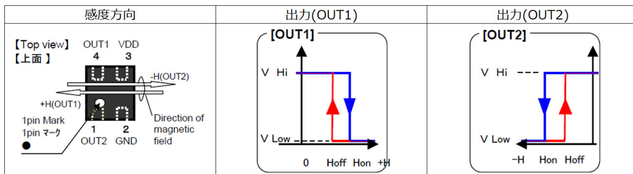
図 1 磁気スイッチ感度方向
