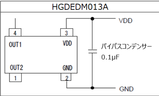
図 6 磁気スイッチ推奨回路
