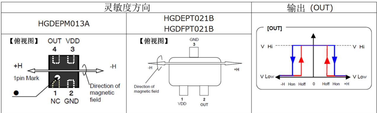
图 1 磁开关灵敏度方向
