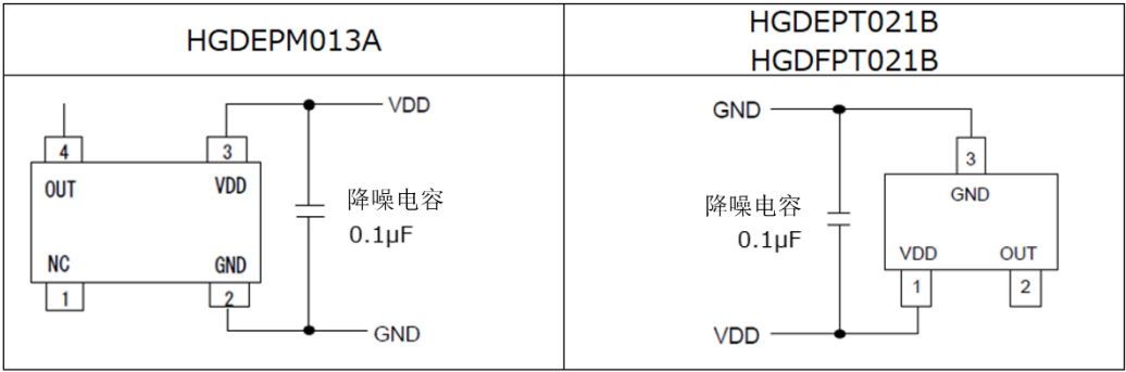
图 6 磁开关推荐电路
