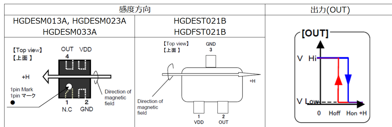
図 1 磁気スイッチ感度方向
