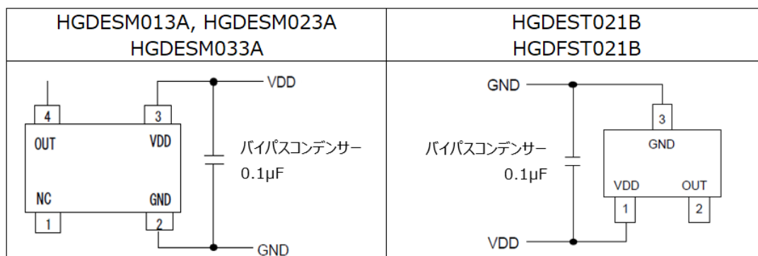
図 6 磁気スイッチ推奨回路
