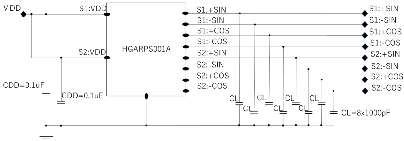
图 7. 磁角度传感器推荐电路
