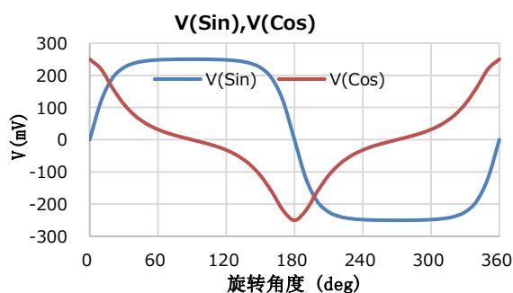
图 15. 传感器输出
