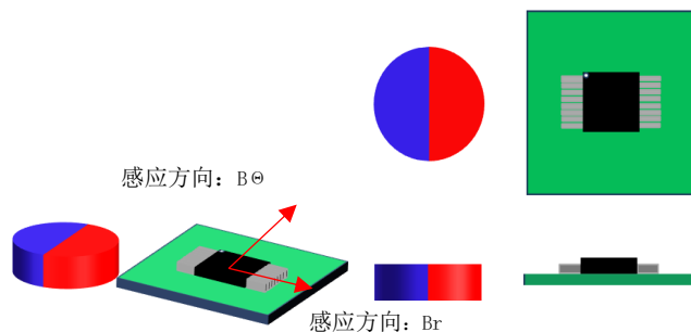
图 13. 磁铁摆放
