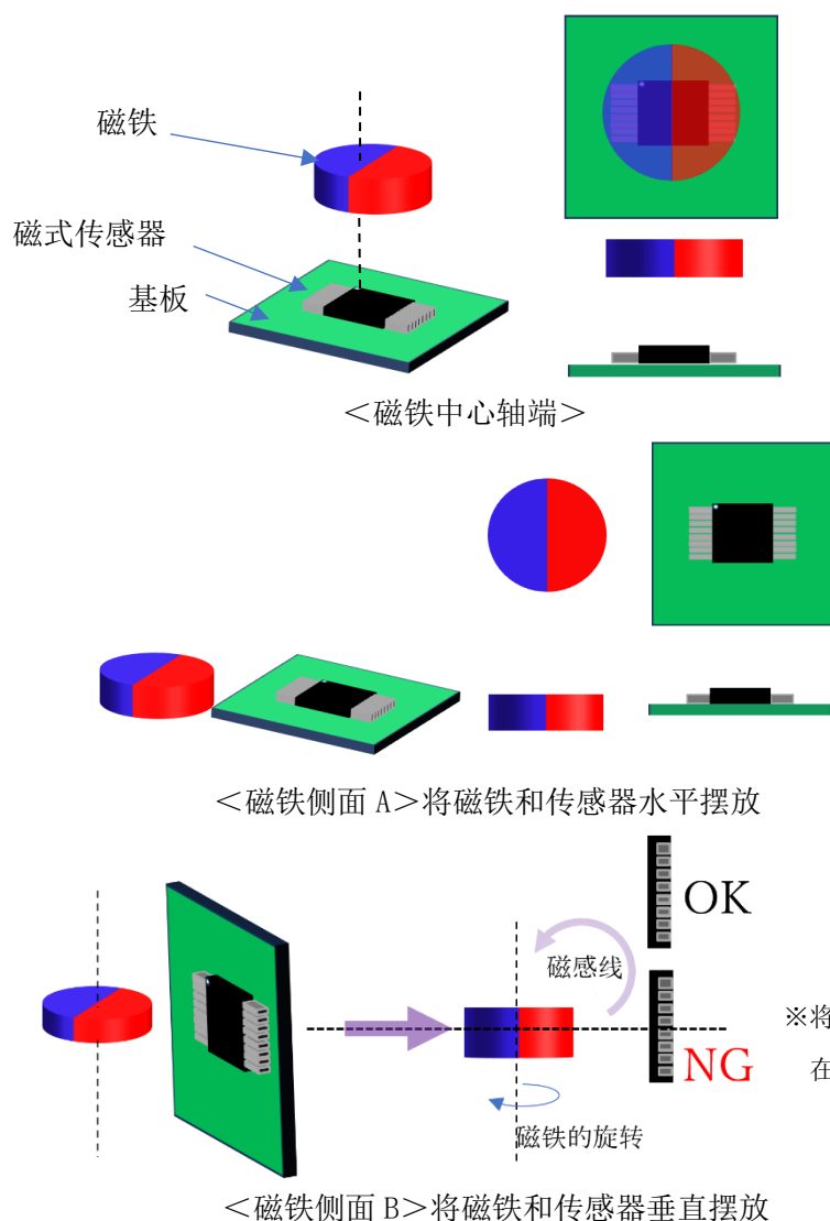
图 5. 磁角度传感器的摆放
