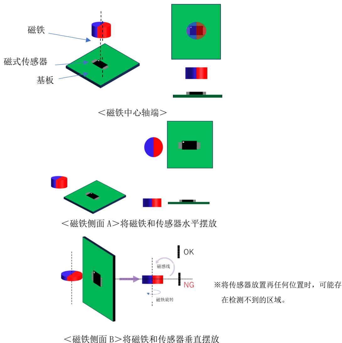
图 5. 磁角度传感器的摆放
