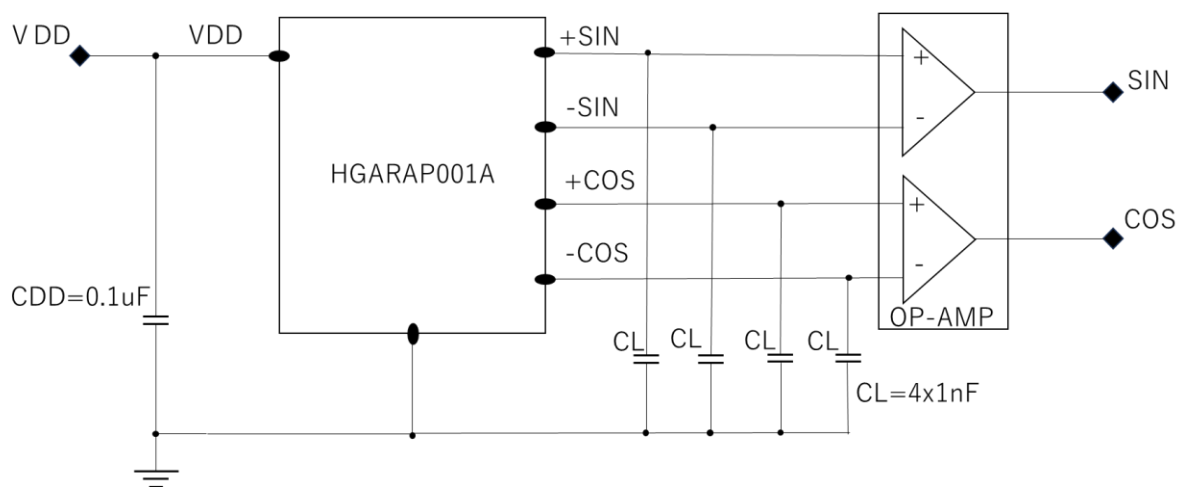
图 7. 磁角度传感器推荐电路
