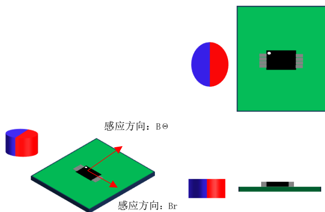
图 13. 磁铁摆放
