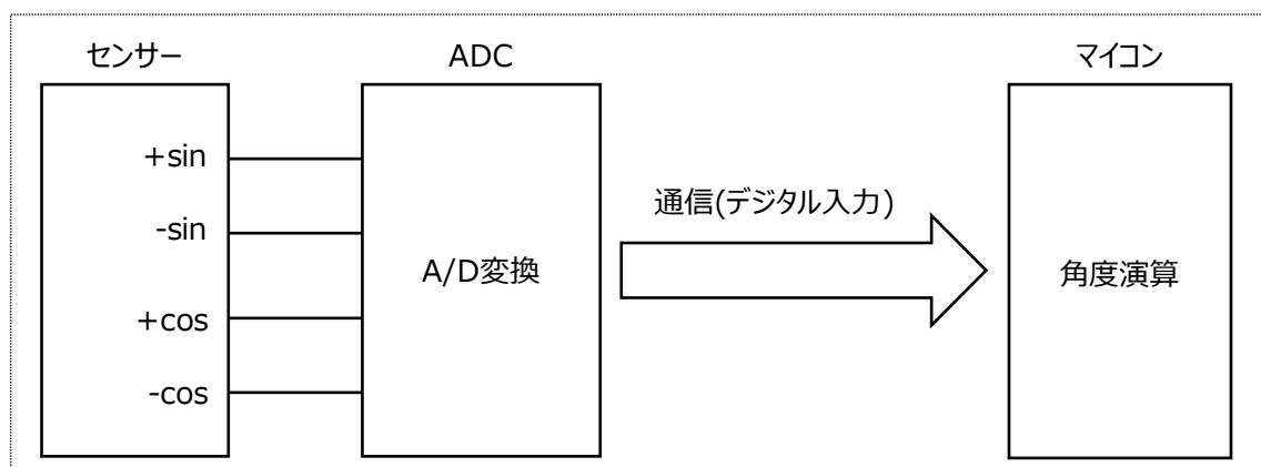
図 3. システム構成例
