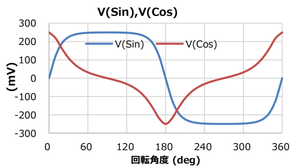
図 15. センサー出力
