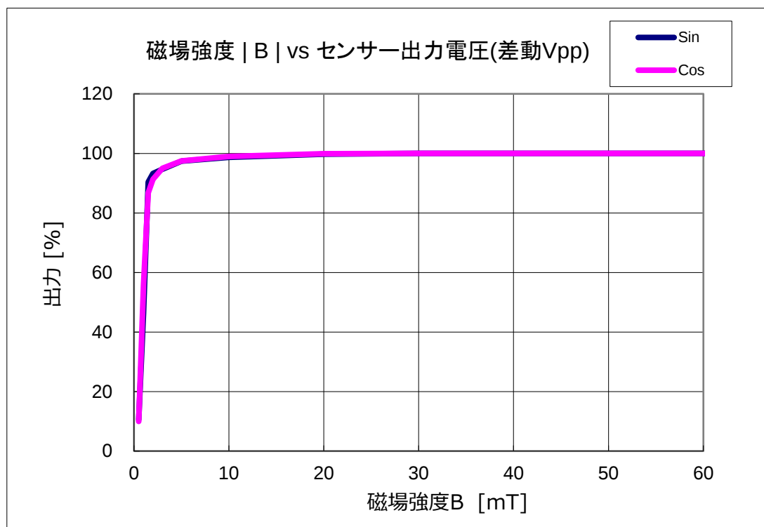
図 6. センサーの出力特性(@VDD 5V)
