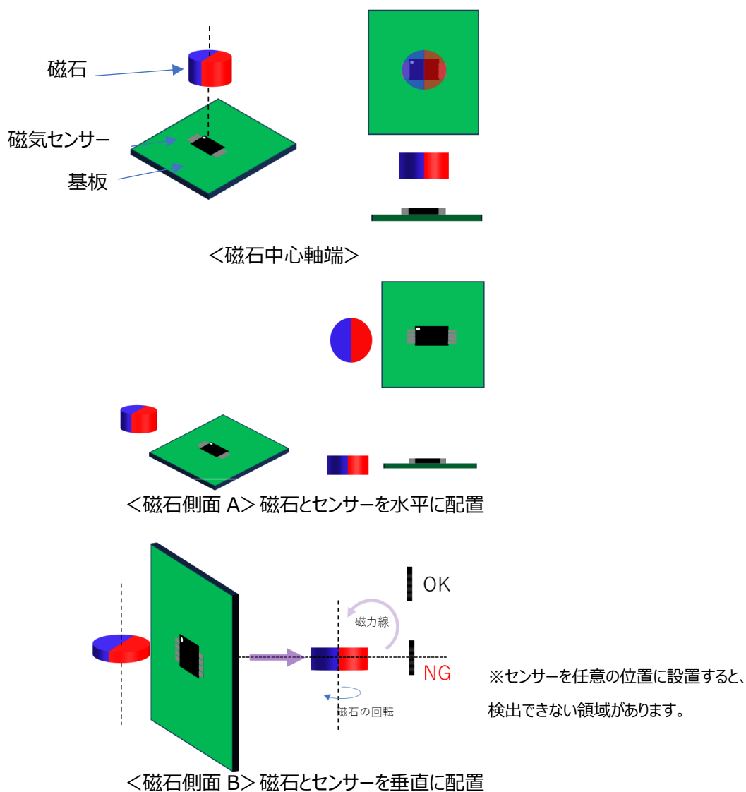
図 5. 磁気角度センサーのレイアウト
