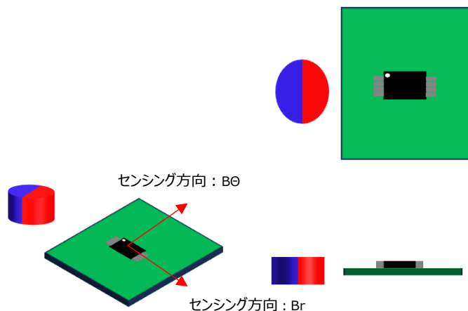
図 13. 磁石のレイアウト
