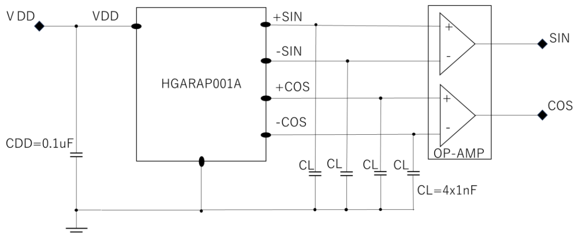
図 7. 磁気角度センサー推奨回路
