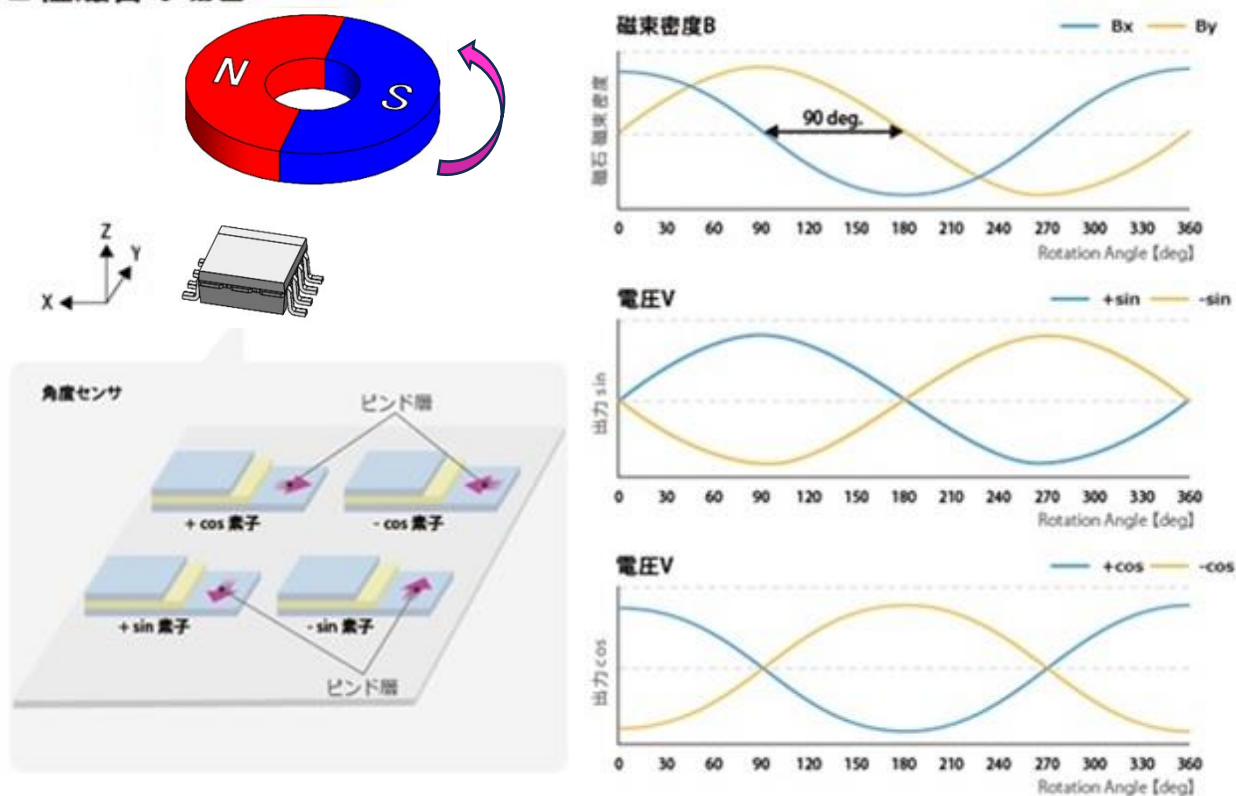
図 1. 磁気角度センサーの出力信号
