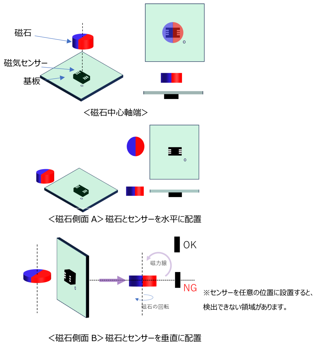
図 5. 磁気角度センサーのレイアウト
