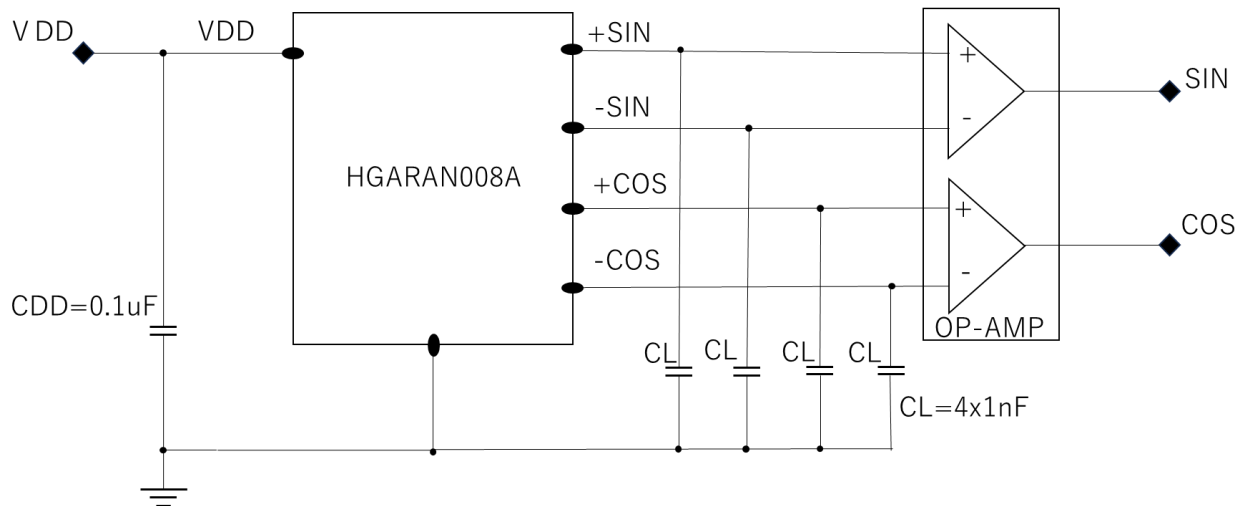
図 7. 磁気角度センサー推奨回路
