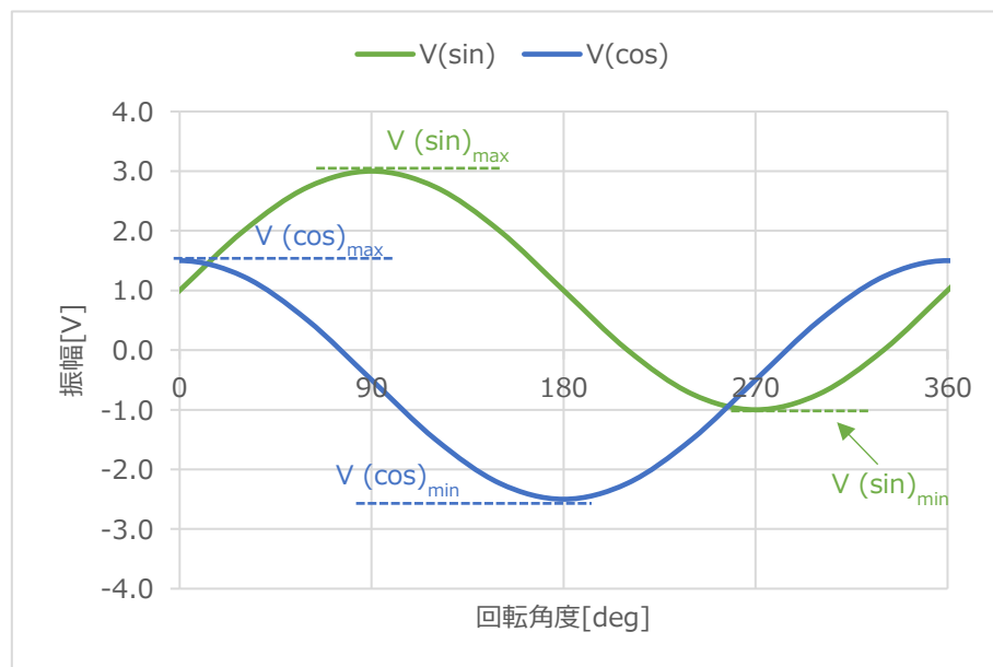
図 21. sin、cos 信号の最大最小値
