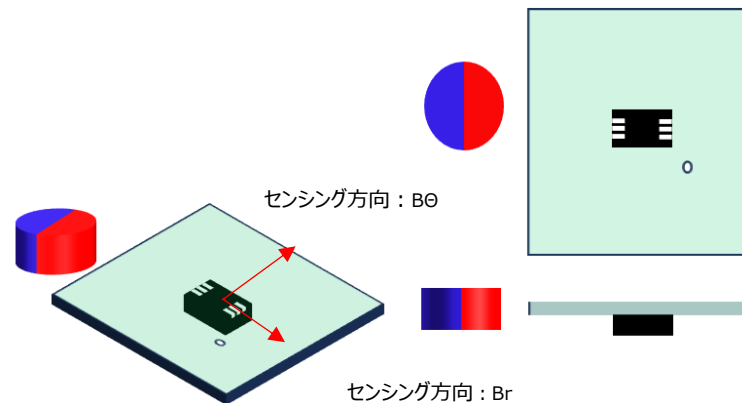
図 13. 磁石のレイアウト
