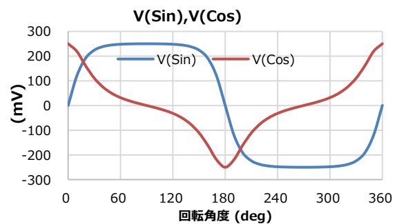
図 45. センサー出力
