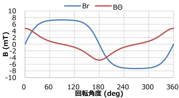
図 34. 磁石の横にある磁場フィールド( B_r , B_\theta )
