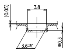
A-A断面図
