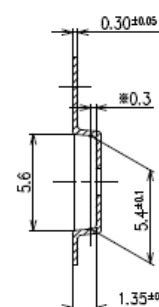
B-B断面图
