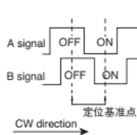
A 相及 B 相均可实现输出规定的示例
