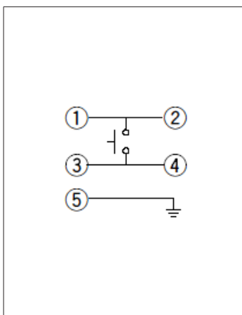
■ 电路图
